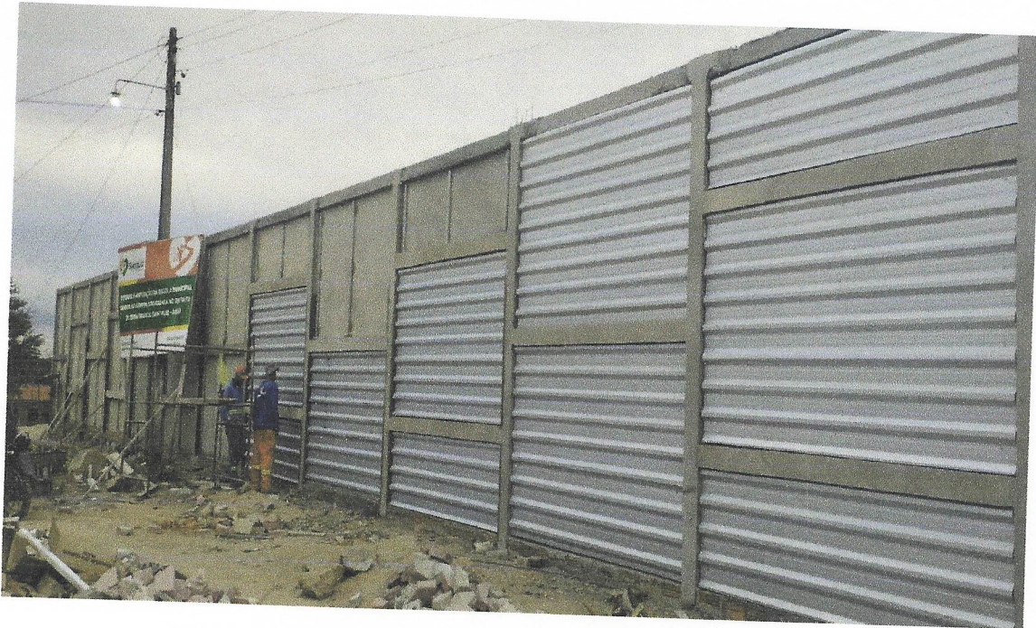
FOTO 25 INSTALAÇÃO DE TELHA METALICA NO MURO FRONTAL
