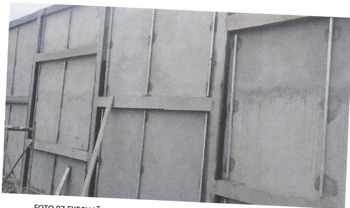
FOTO 07 EXECUÇÃO DE FIXADOR PARA INSTALAÇÃO DAS TELHAS METALICAS
